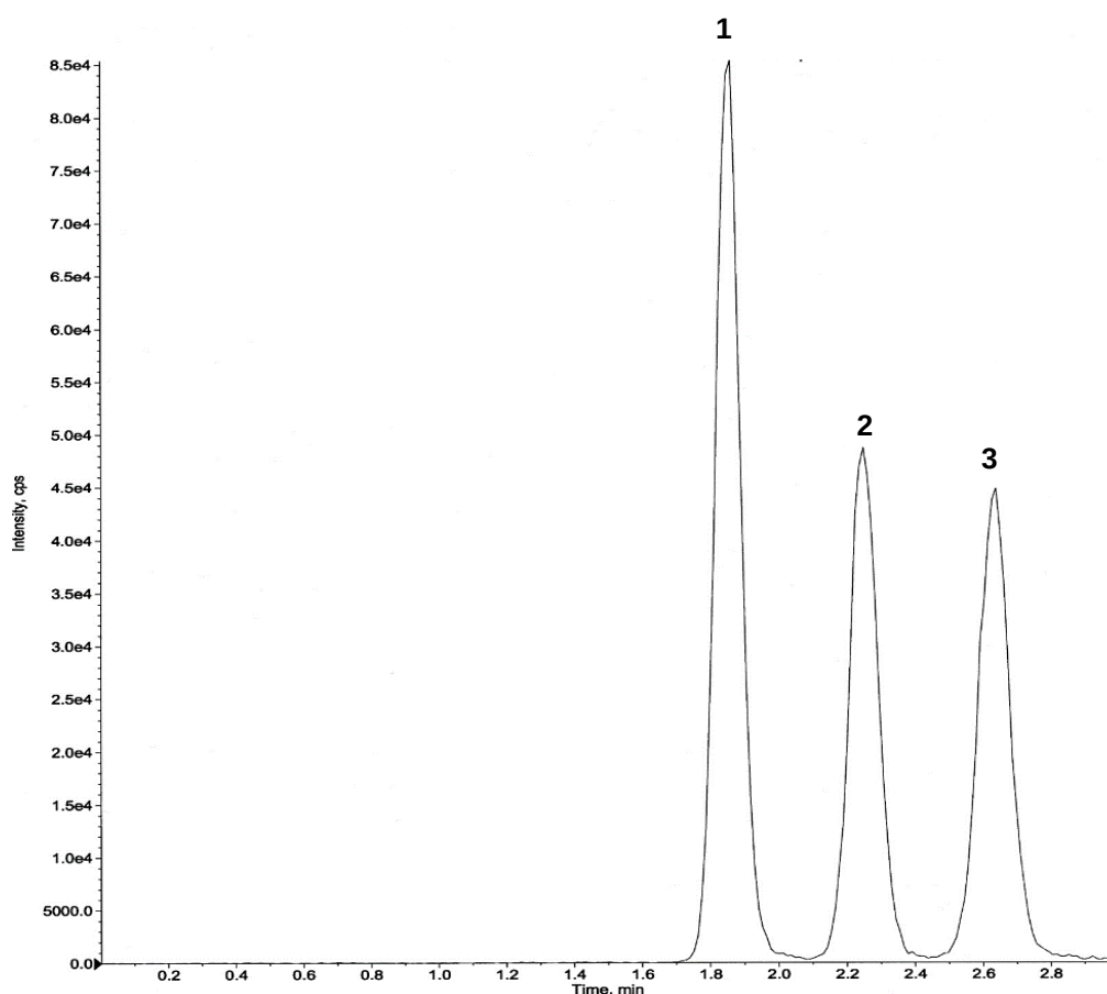
1. 6-epi-Pravastatin (MW: 424)
