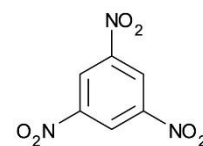
1. 1,3,5-Trinitrobenzene
