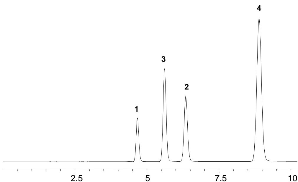
1. 1,3,5-Trinitrobenzene
