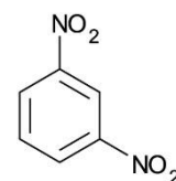
3. 1,3-Dinitrobenzene
